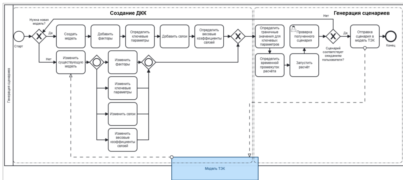
Рис. 1. Моделирование процесса генерации сценариев
