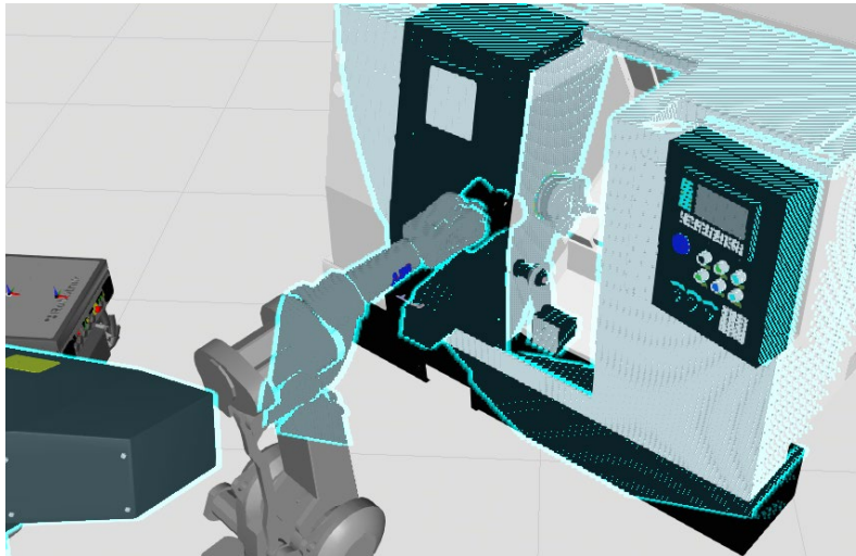
Рис. 3. Пример визуализации работы RGB-D камеры в модели РТК
