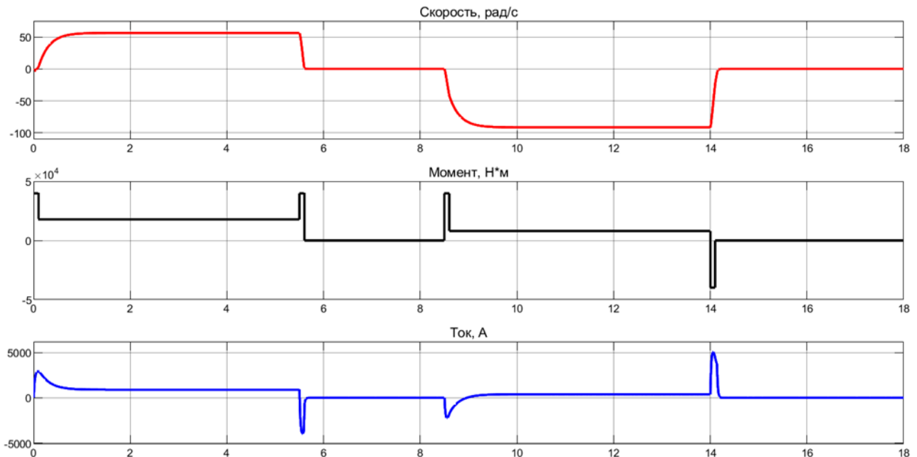
Рис. 5. Переходные процессы в модели электропривода механизма подъема ковша шагающего экскаватора с частотно-импульсным управлением
