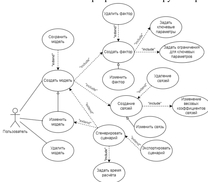
Рис. 2. Функциональные возможности приложения
