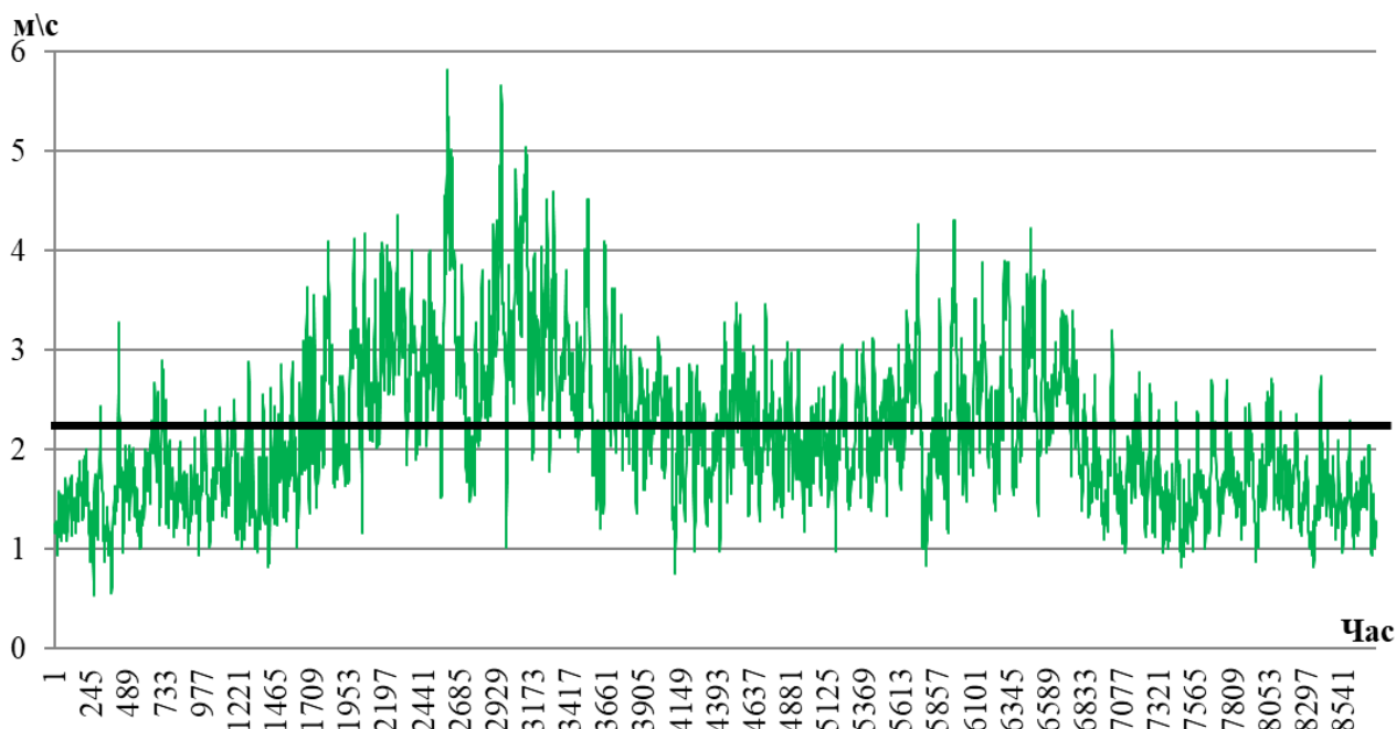
Рис. 2. Расчетные значения скорости ветрового потока в течение года на высоте 10 м (высота метеостанции)
