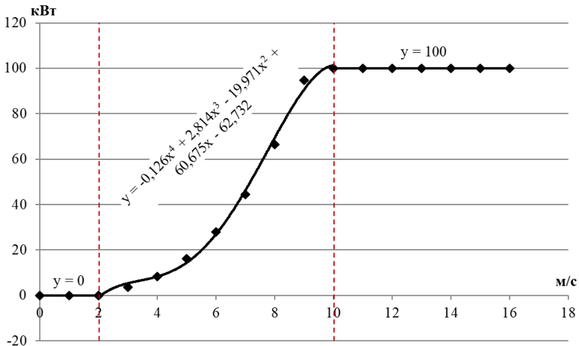
Рис. 5. Аппроксимация кривой развиваемой мощности ВЭУ методом сплайнов
